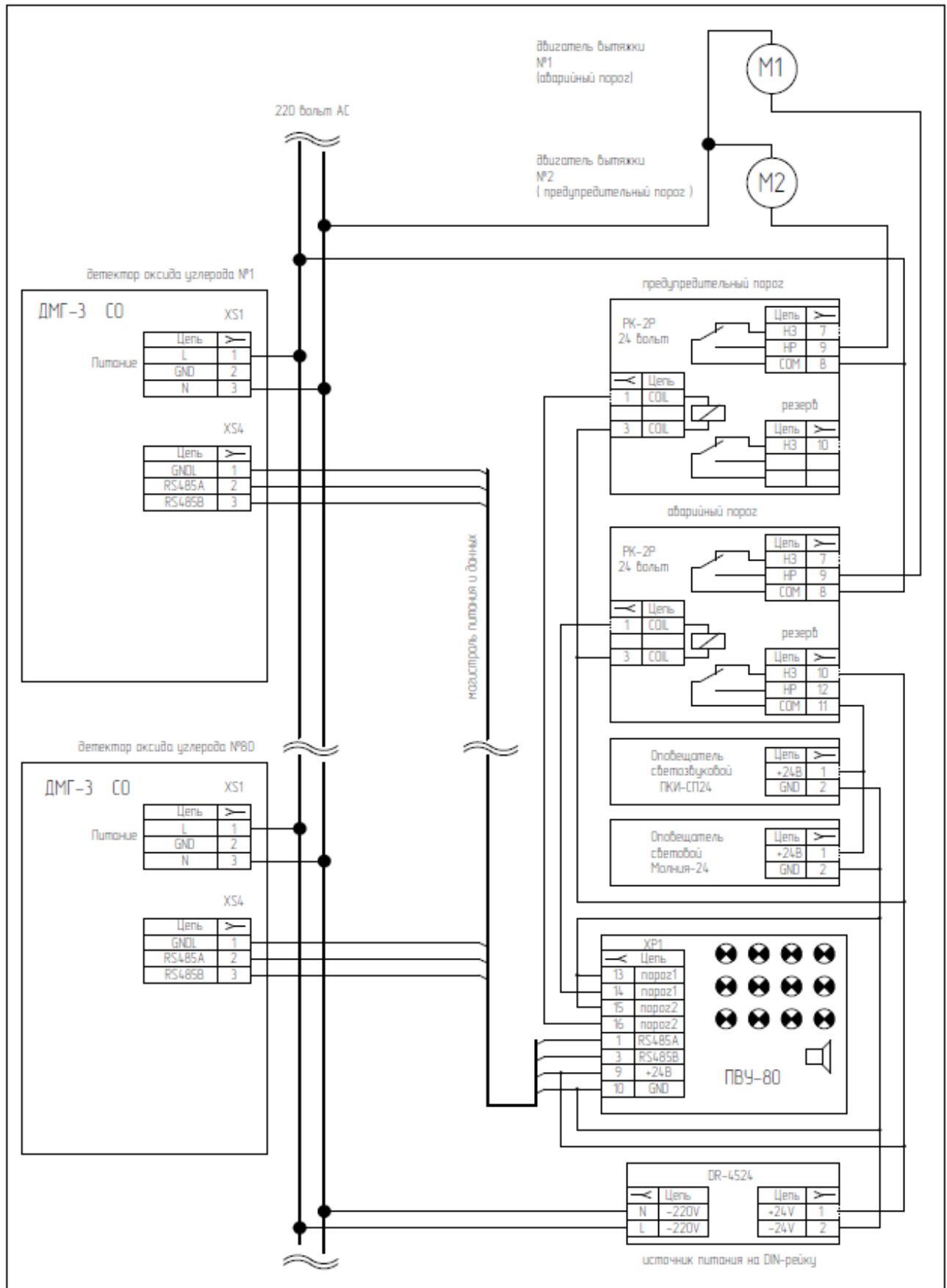
Рисунок А.2 – Структурная схема изделия с детектором контроля оксида углерода ДМГ-3
